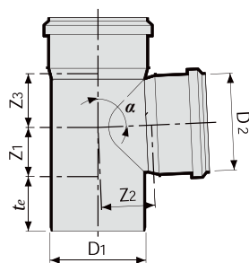
Тройник
