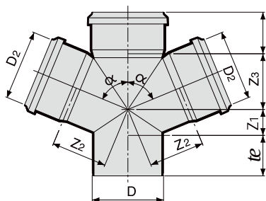
Крестовина
